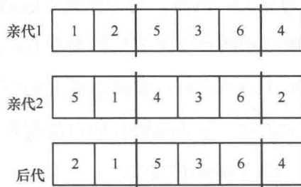
图 4-3 排序交叉示例
