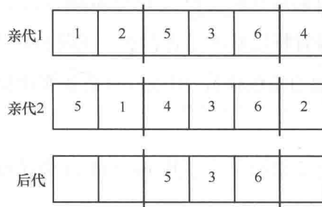
图 4-2 排序交叉
