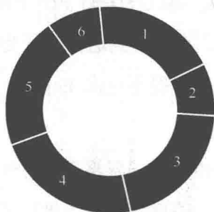
图 2-1 轮盘赌
