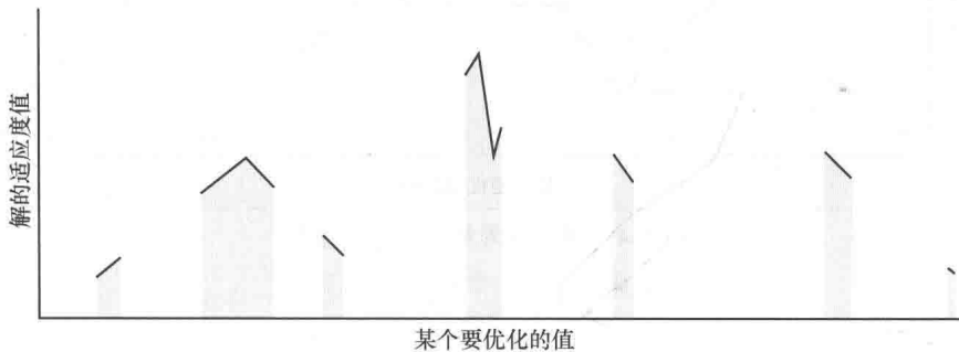
图 1-2 更典型的适应度空间搜索
