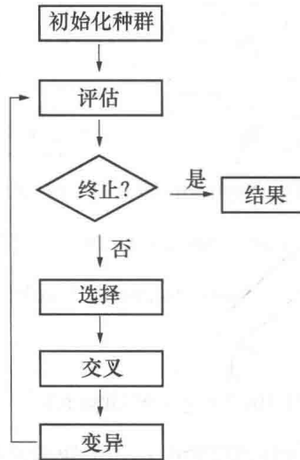
图 1-10 一般遗传算法的过程
