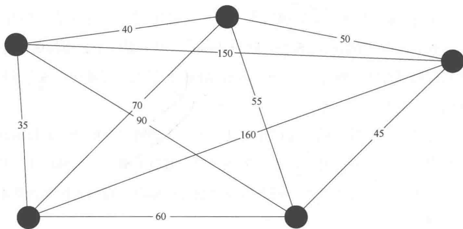
图 4-1 城市和它们之间的距离
