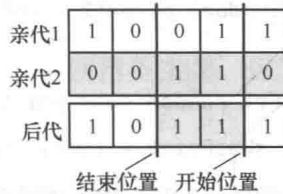
图 3-5 两点交叉
