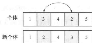
图 4-4 交换变异
